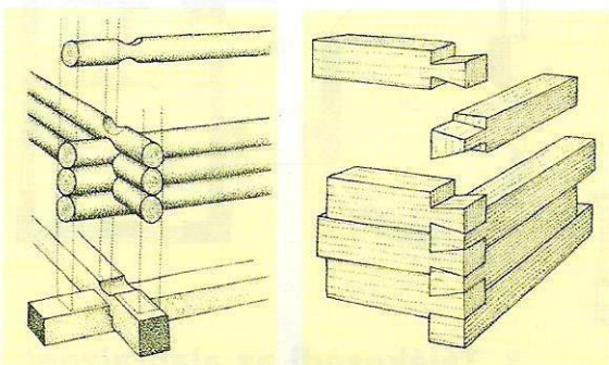
A boronafal építésének típusai
